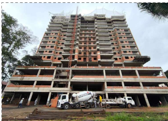
FOTO 3 – Concretagem dos pilares da cobertura do 15º Pav
